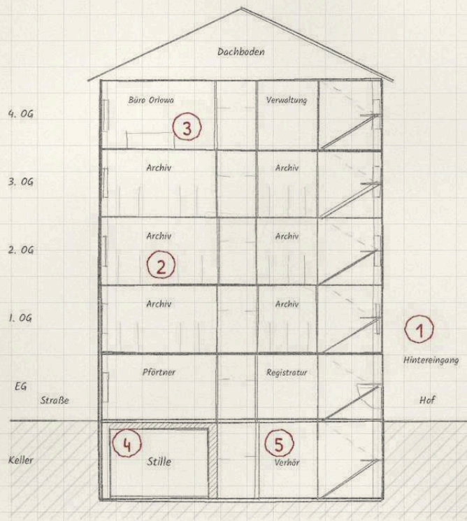
Querschnitt
