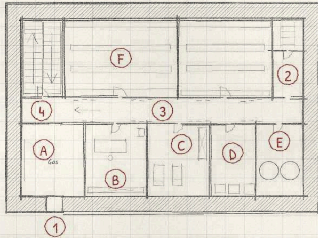
2. Obergeschoss
