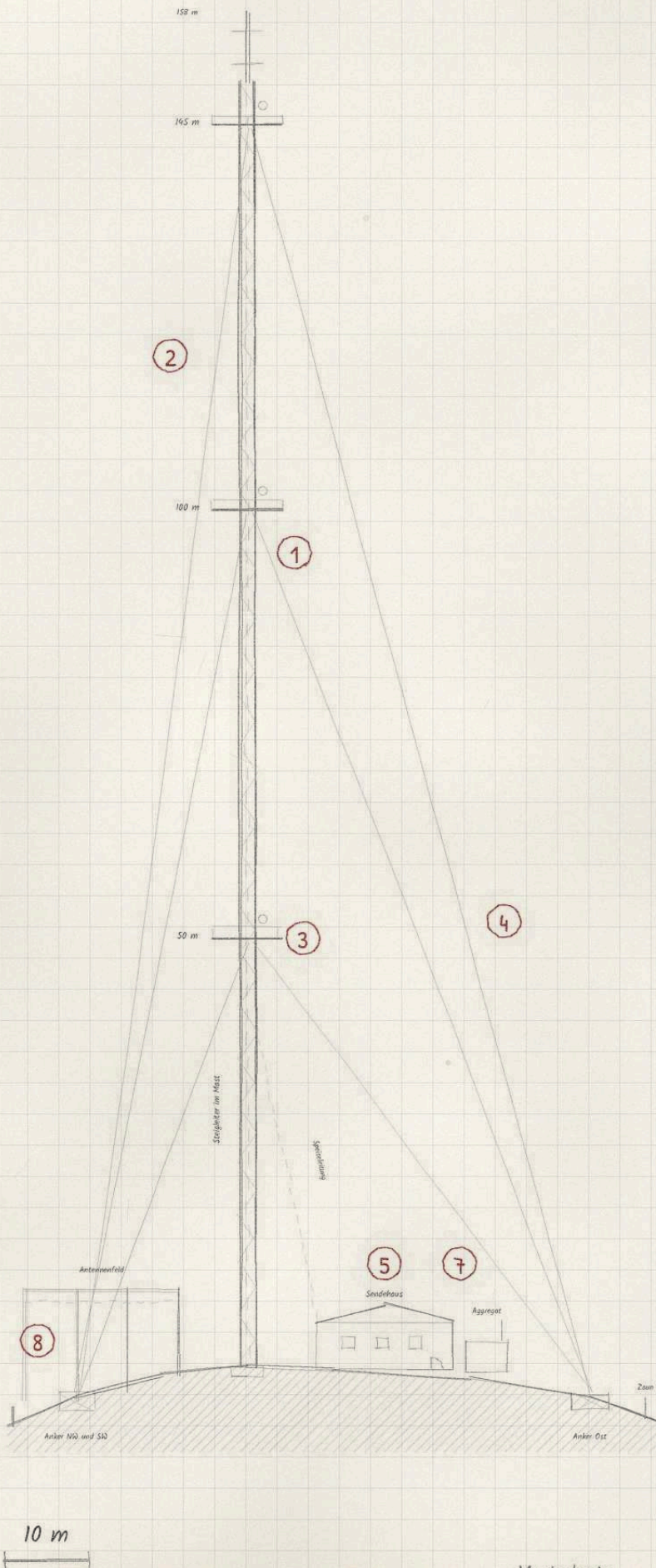
Ansicht von Süden
