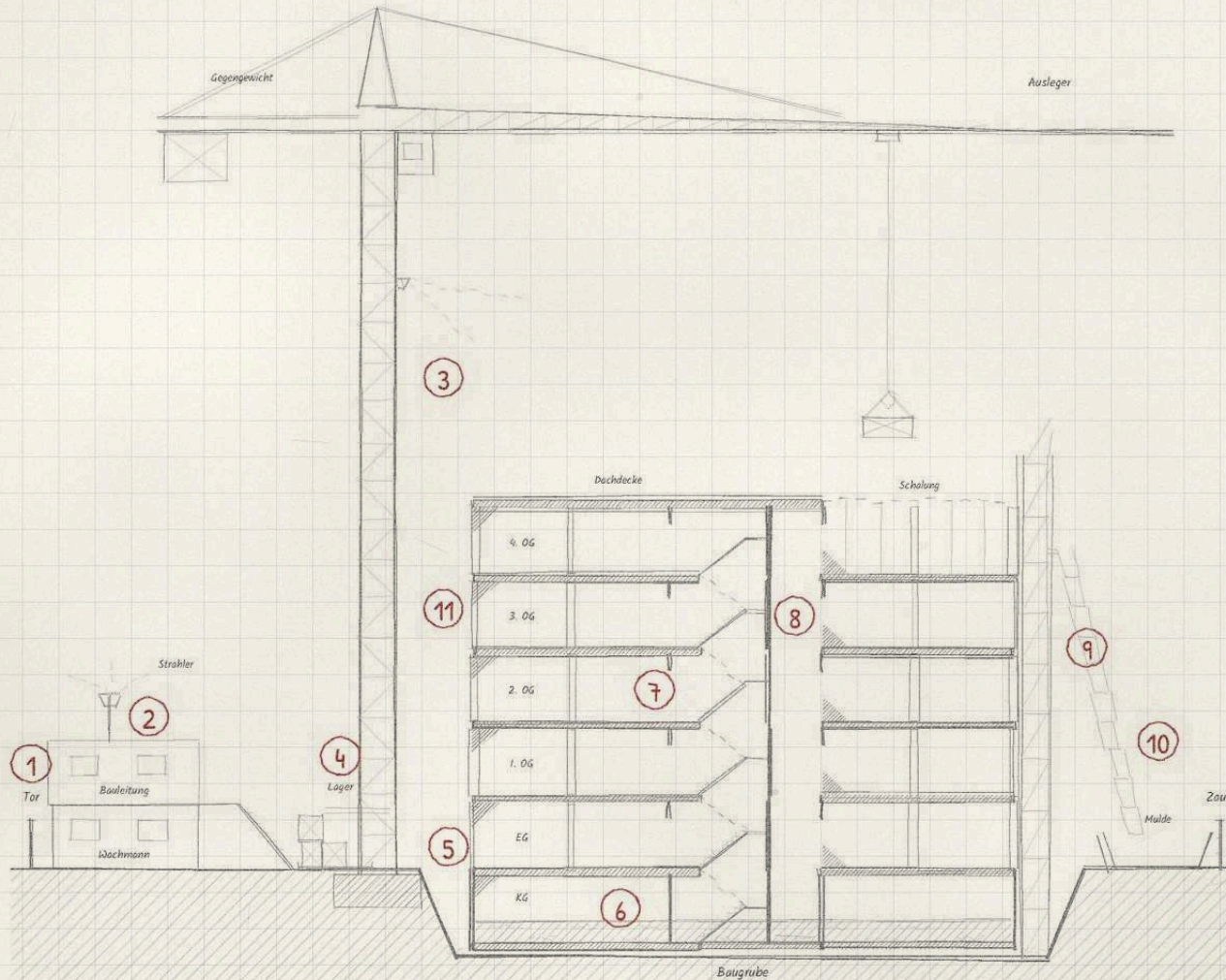
Querschnitt, Blick nach Norden
