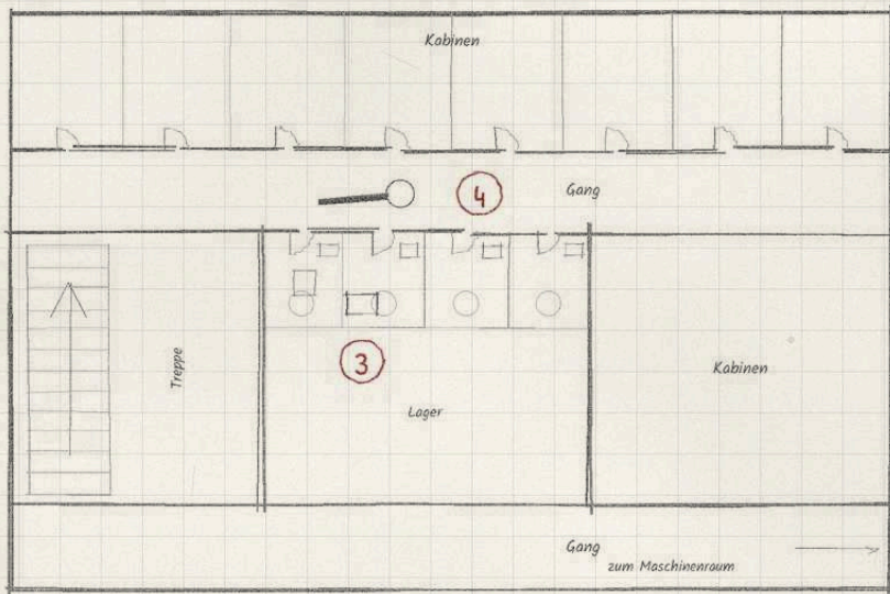
Zwischendeck, Ausschnitt, etwa doppelt so groß
