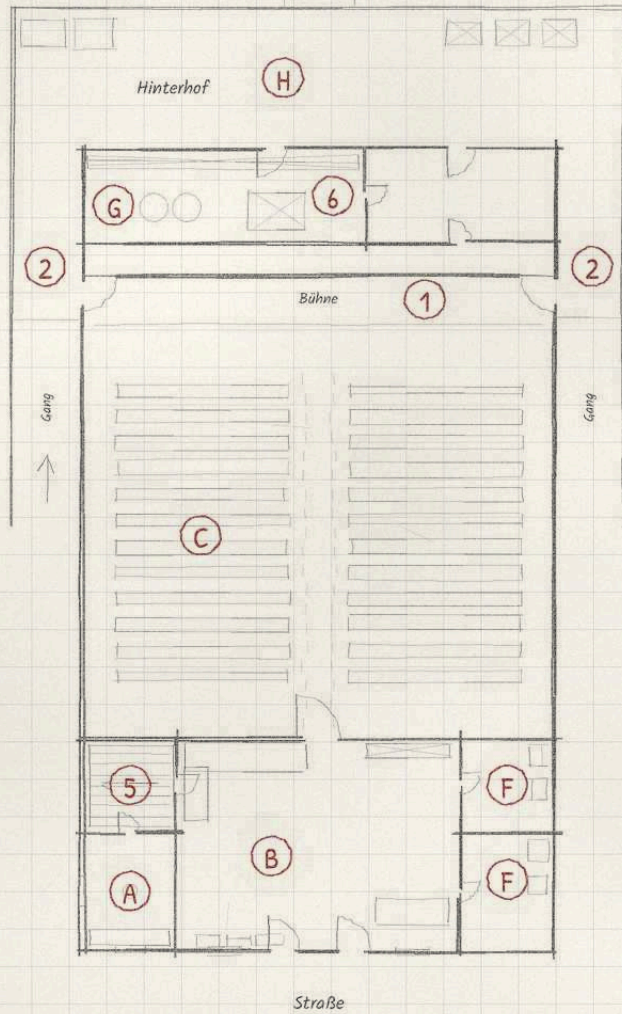
Erdgeschoss
