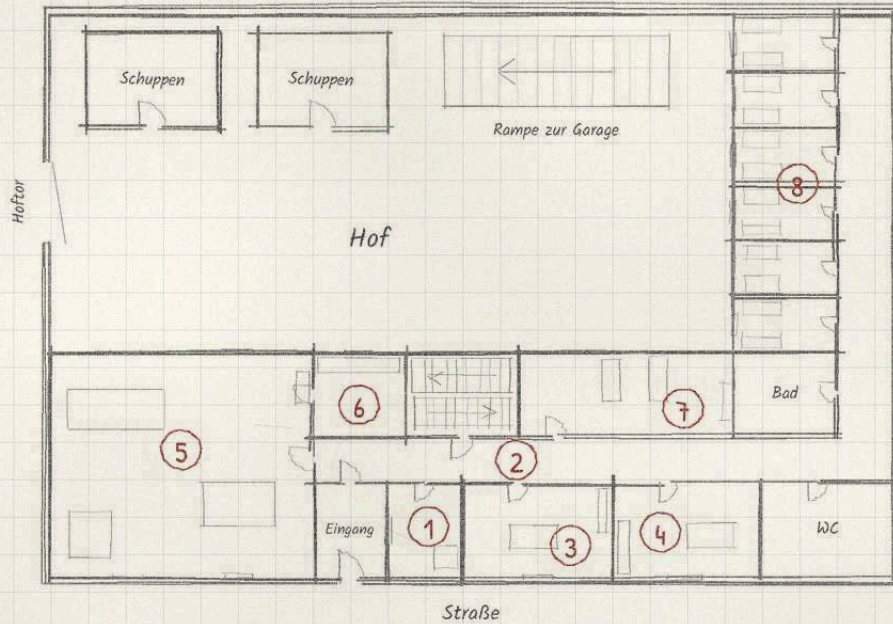
Ebene 0, Erdgeschoss
