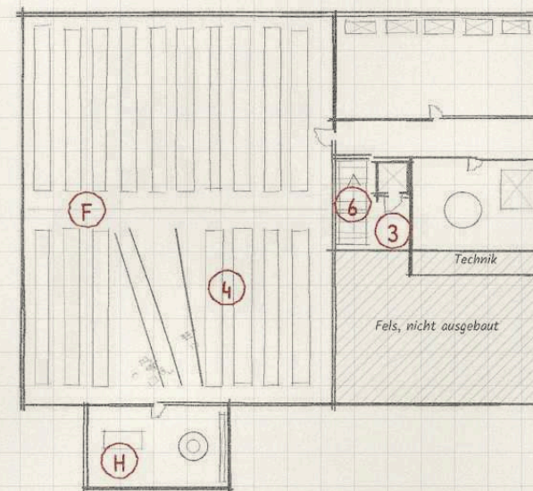
2. Untergeschoss, unteres Magazin
