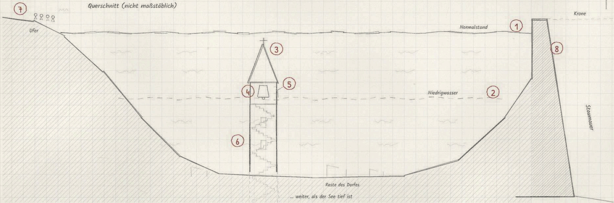
Lageplan Ufer
