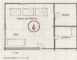
Sendehaus, Grundriss
