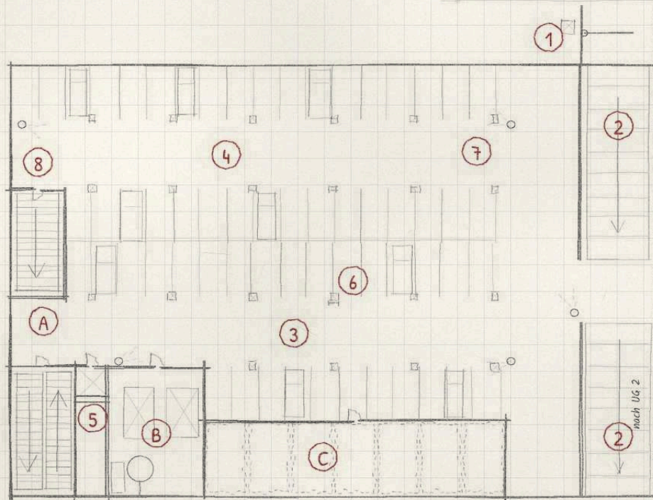
Untergeschoss 1
