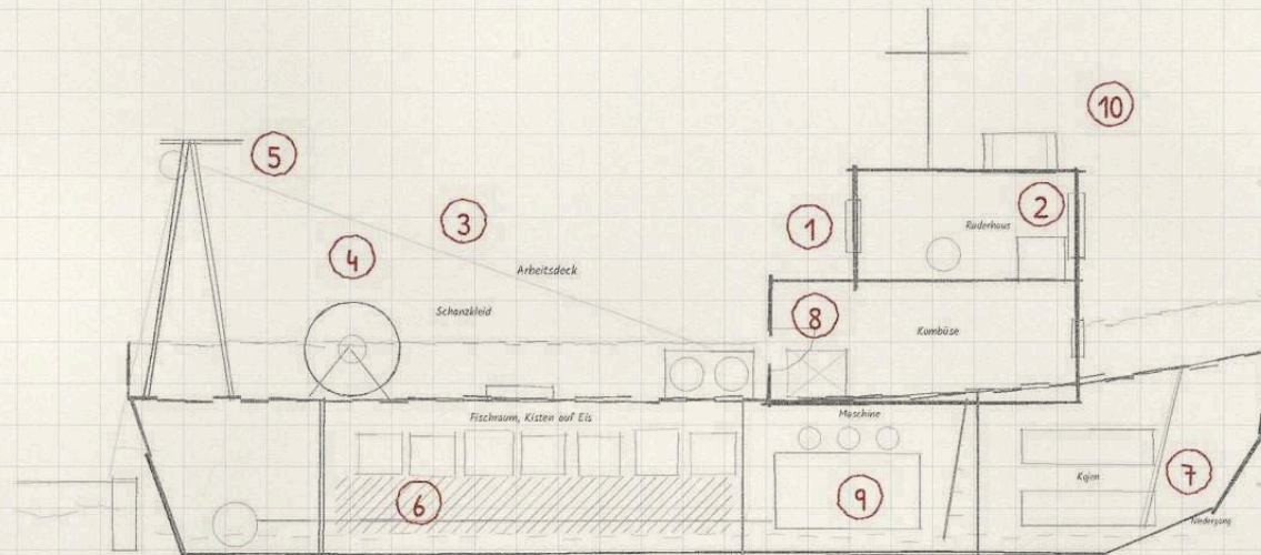
Längsschnitt, Bug rechts
