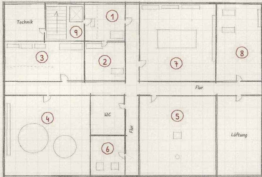
Ebene A, Arbeitsebene
