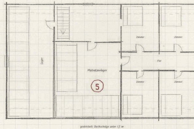
Dachgeschoss
