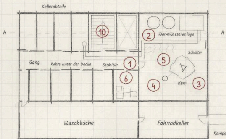
Grundriss Keller
