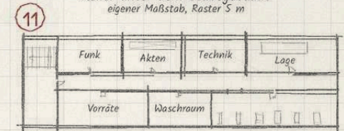
Keller unter dem Stabsgebäude eigener Maßstab, Raster 5 m
