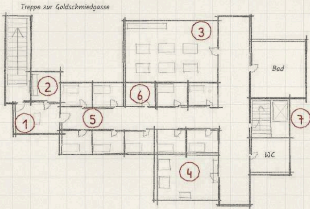
UG 1, Wohngeschoss
