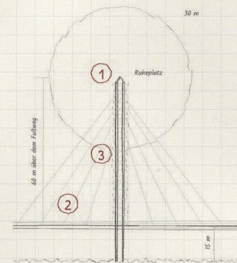
Pylon Nord, Ansicht, 2,5-fach
