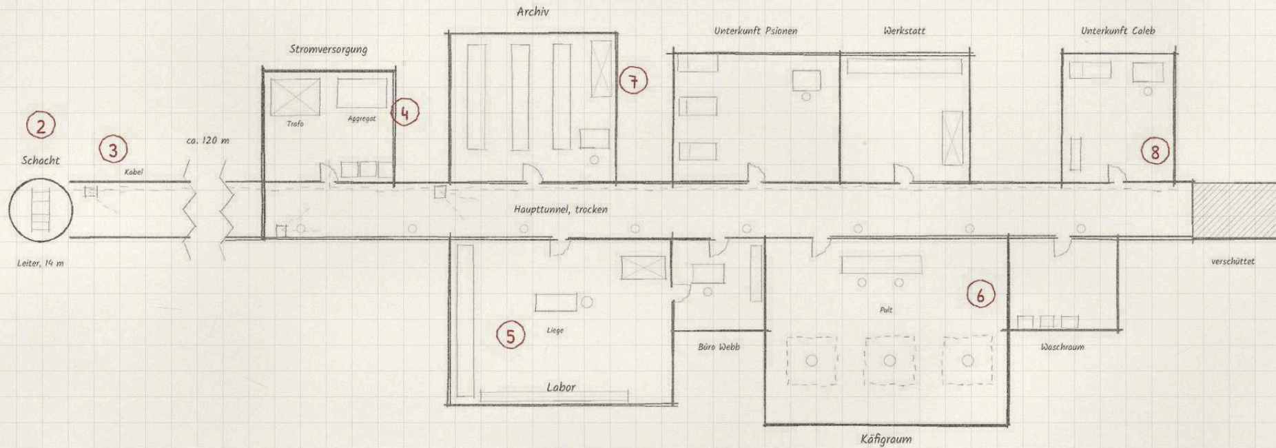
Nebenfeld: Lageplan des Reservoirs (eigener Maßstab)
